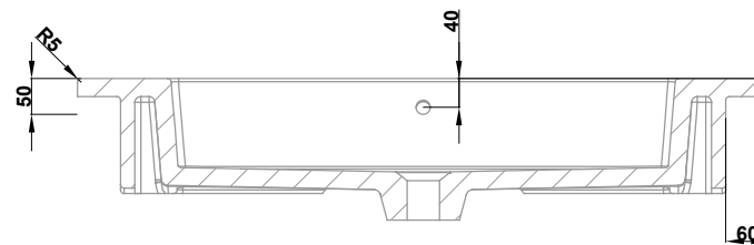
SEZIONE B-B
